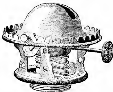
Fig. 3377. "UNIQUE" SUN-HINGE BURNER. (Sun-hinge Chimney, Nos. 14 and 17.)
